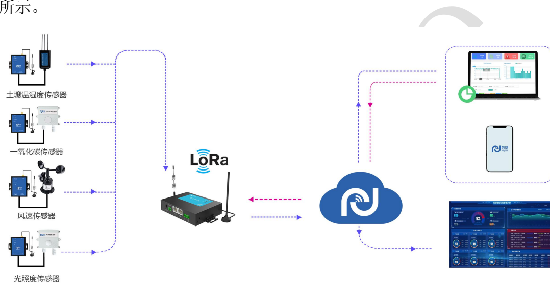
系统框架图
