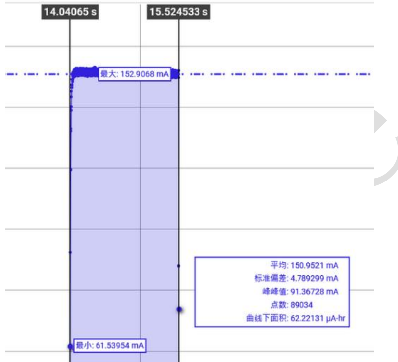
上报数据电流消耗（SF12）
